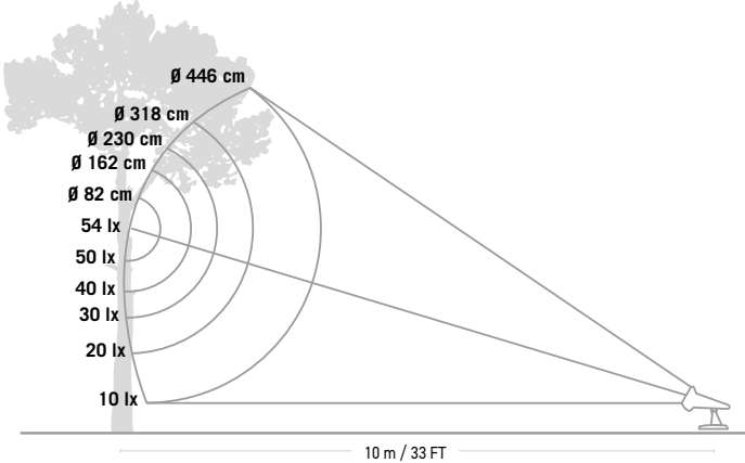
LUX /DISTANCE pour une implantation à 10 m LUX /DISTANCE form a position 33 FT away
