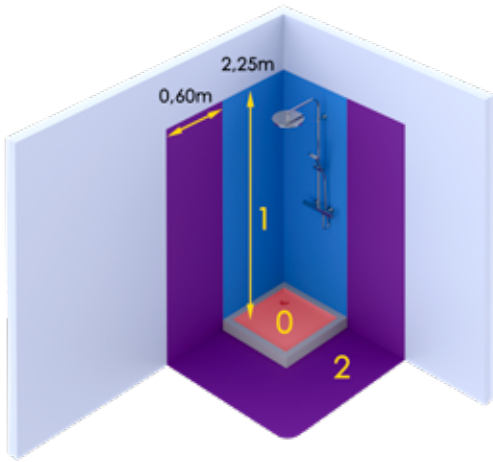
CAS 2 Exemple de local contenant une douche avec receveur
