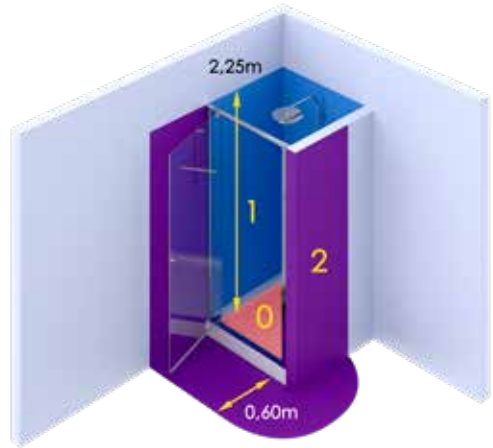
CAS 4 Exemple de local contenant une douche avec receveur et une paroi murale
