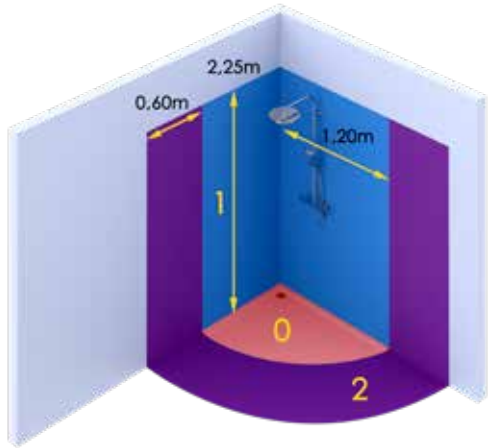
CAS 3 Exemple de local contenant une douche sans receveur
